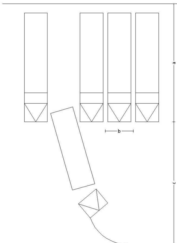
ΑΠΑΙΤΟΥΜΕΝΟΣ ΧΩΡΟΣ ΚΑΘΕΤΗ ΣΤΑΘΜΕΥΣΗ
