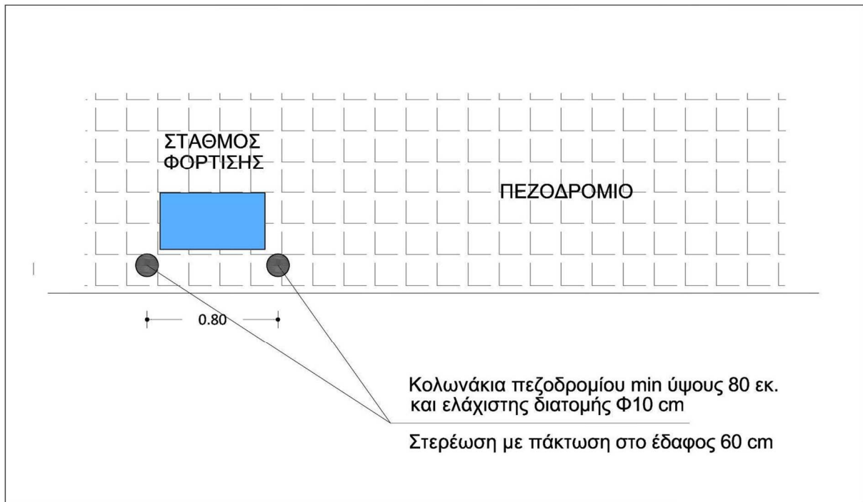
ΘΕΣΕΙΣ ΚΑΤΑ ΜΗΚΟΣ ΣΤΑΘΜΕΥΣΗΣ ΦΟΡΤΗΓΩΝ ΓΙΑ ΦΟΡΤΙΣΗ Η/Ο
