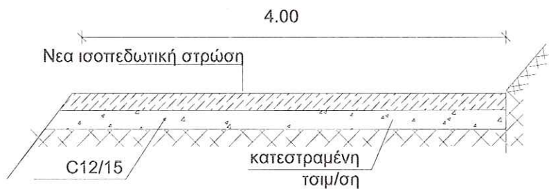
ΤΥΠΙΚΗ ΔΙΑΤΟΜΗ ΟΔΟΥ
